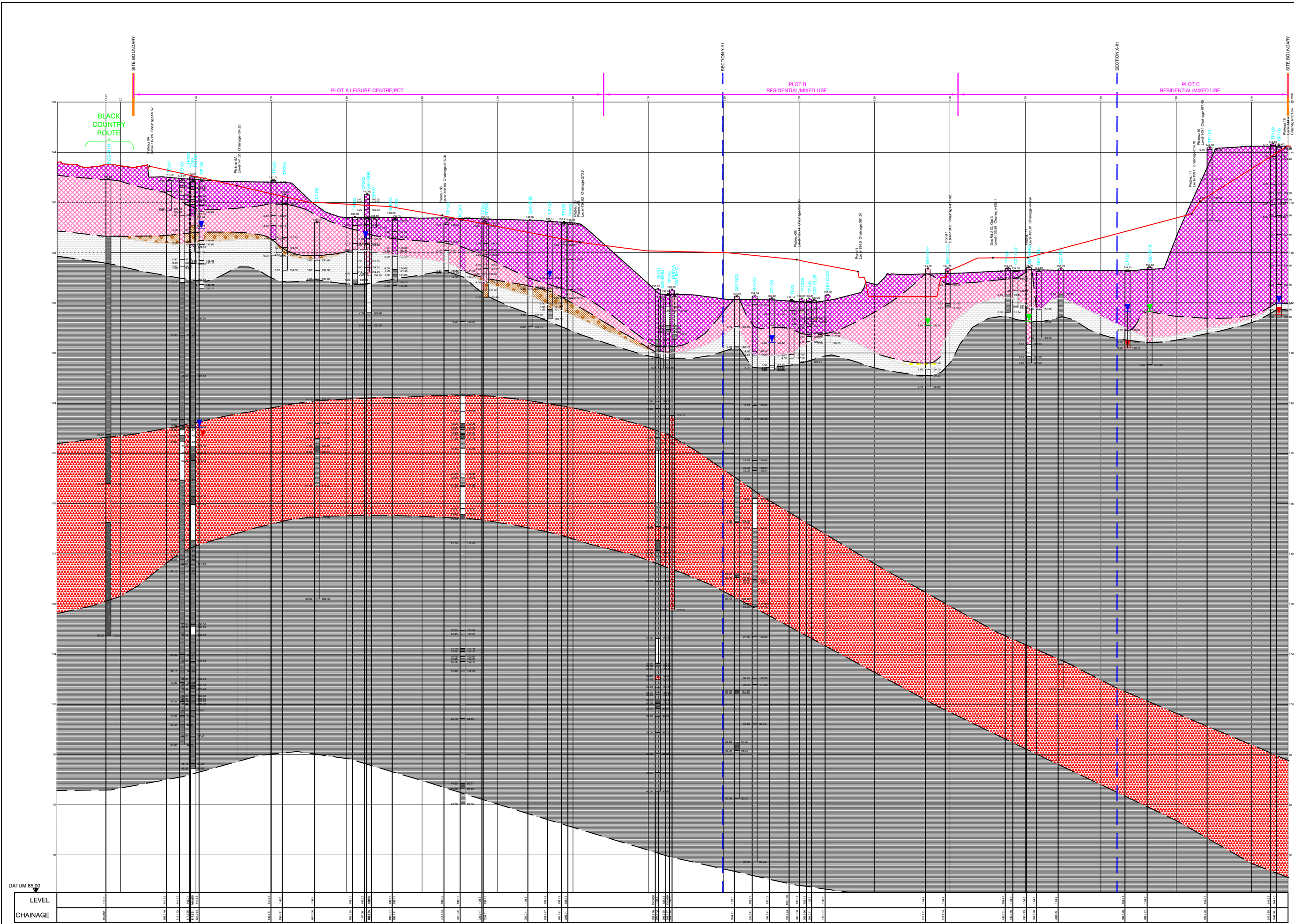
SECTION C-C1 Horiz. 1:500 Vert. 1:100
